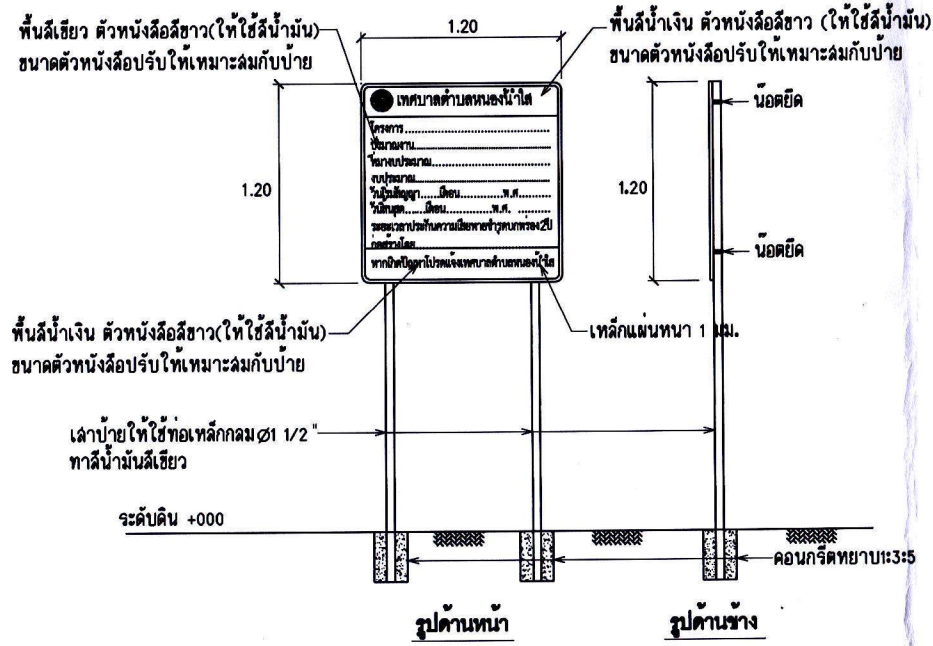
แบบป้ายโครงการ
