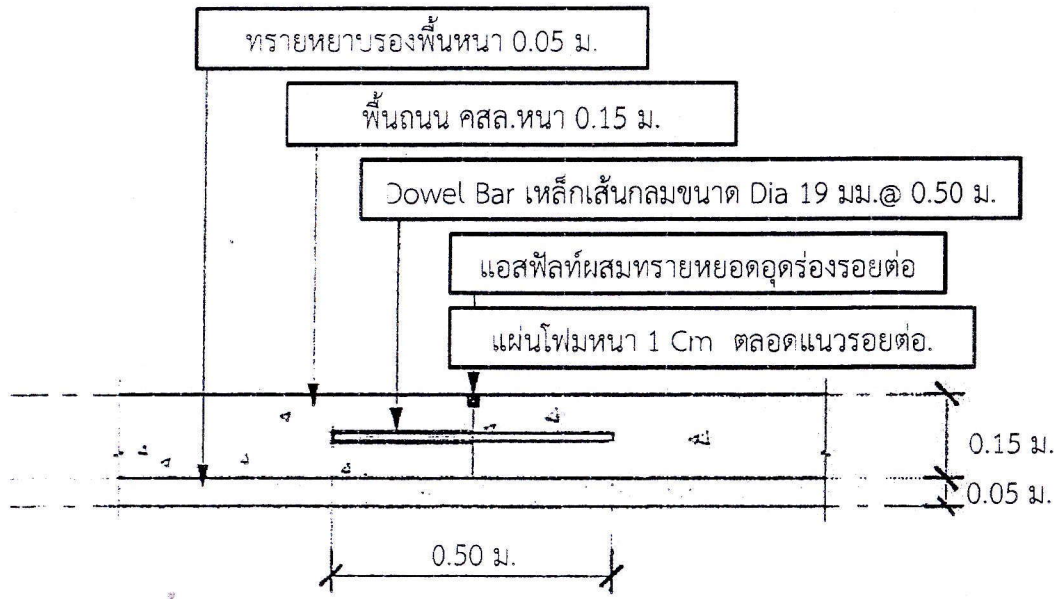
ขยาย expansion joint @ 50.00 ม.
