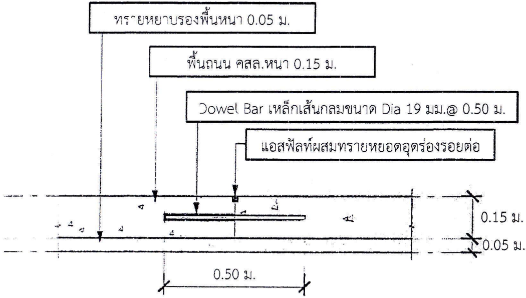
ขยาย Contraction joint @ 5.00 ม.
