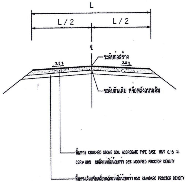
รูปตัด โครงสร้างทาง
