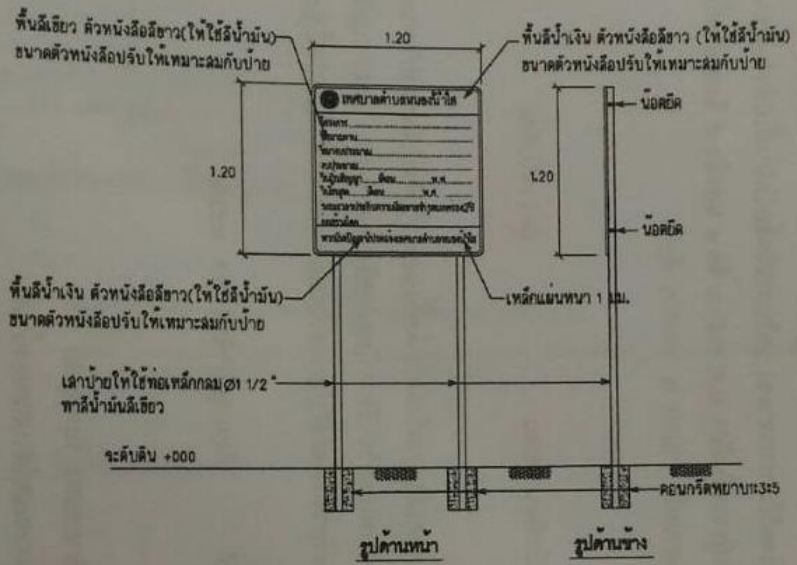
แบบป้ายโครงการ
