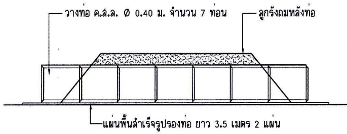
รูปด้านข้างท่อระบายน้ำ
