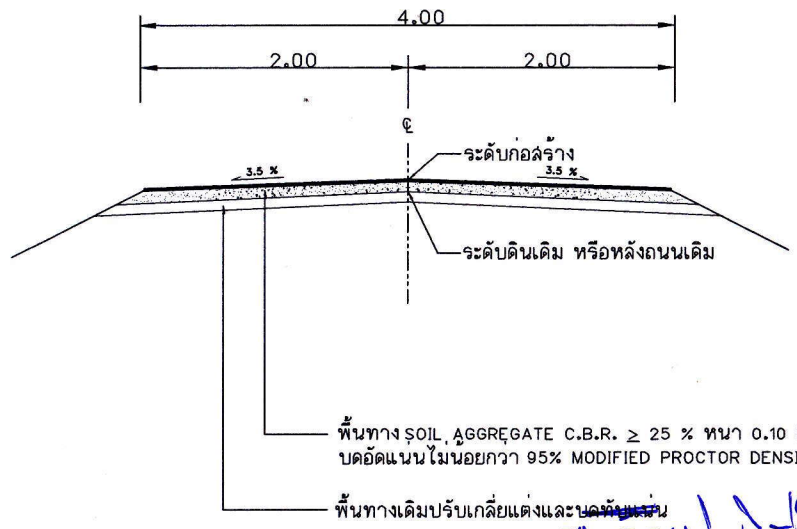
รูปตัดโครงสร้างทาง
