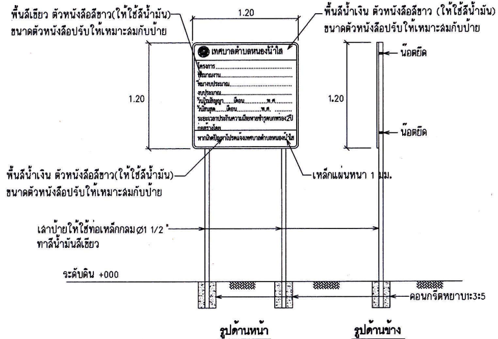
แบบป้ายโครงการ
