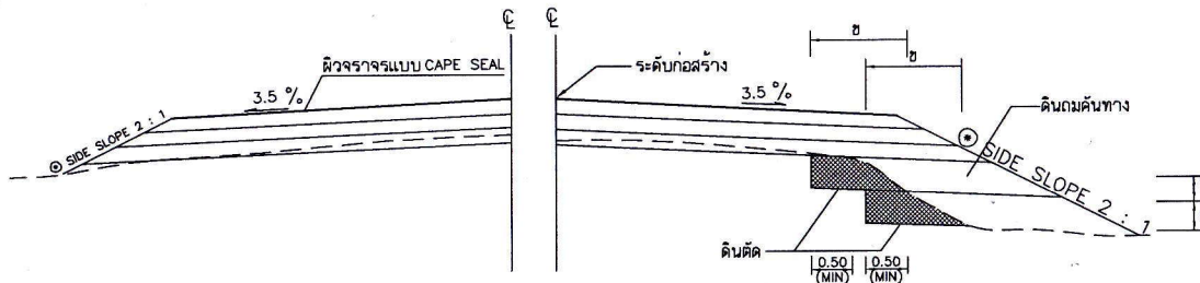
รายละเอียดการก่อสร้าง
