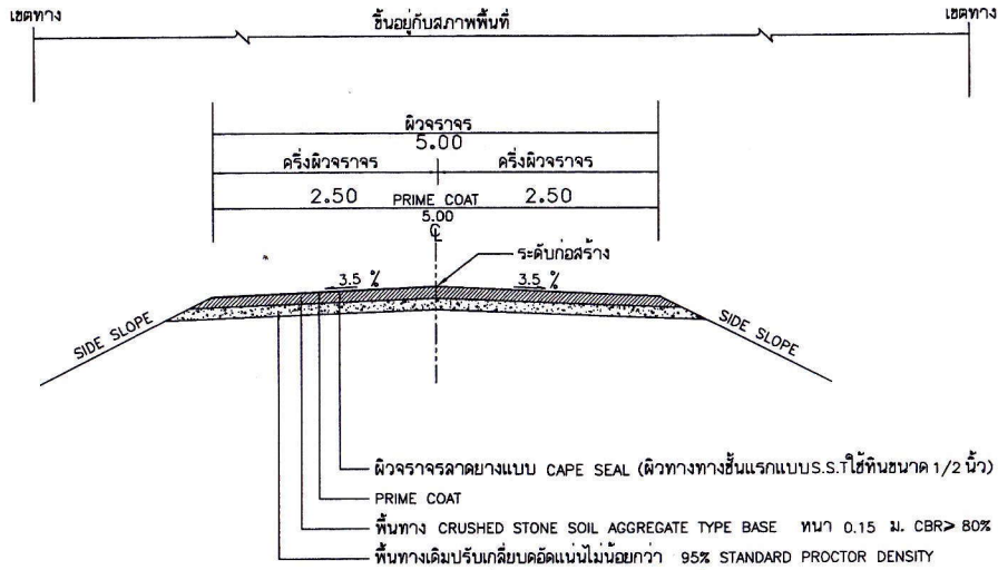
รูปตัดโค้งสร้างทาง
