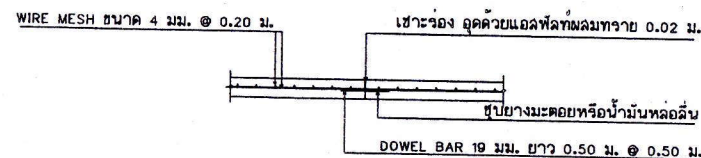
ขยายรอยต่อ CONSTRUCTION JOINT
