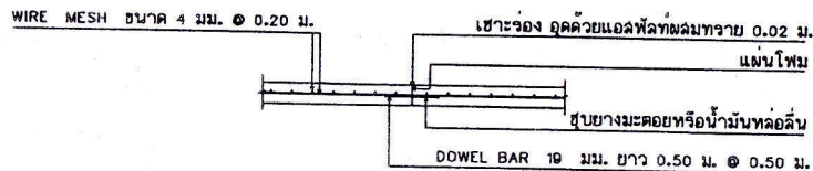
ขยายรอยต่อ EXPANSION JOINT
