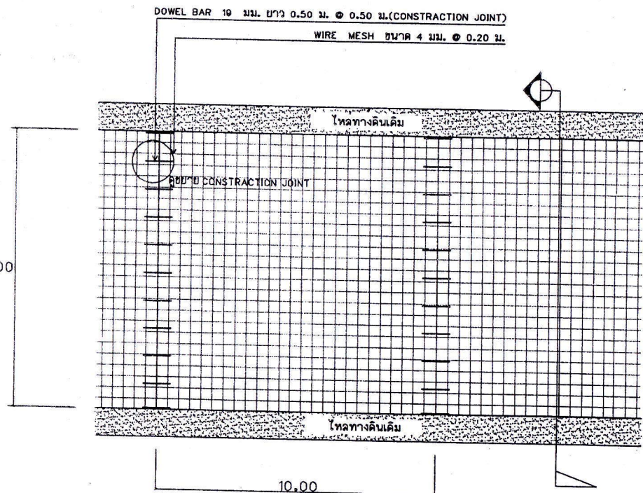
แปลนถนน
