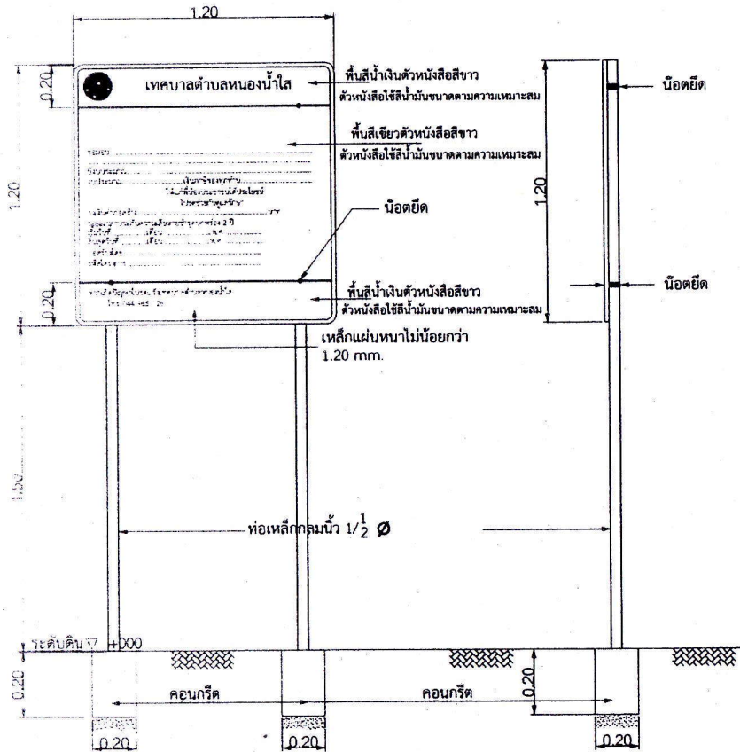
ด้านหน้า ไม่แสดงมาตราส่วน ด้านข้าง ไม่แสดงมาตราส่วน
